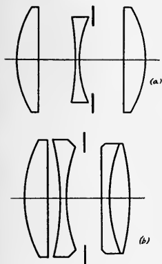
FIG. 2a. Triplet lens.
